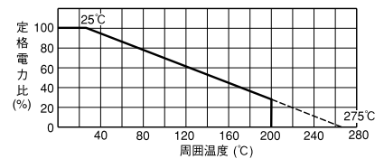
周囲温度と電力軽減曲線
